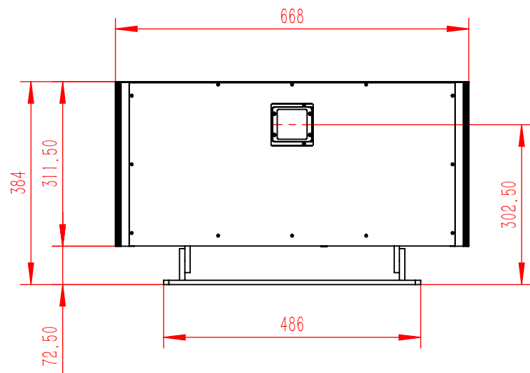
KVANT Spectrum20防水箱尺寸图
